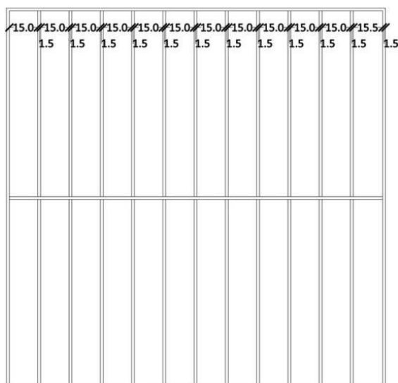
Protecciones metálicas tipo
